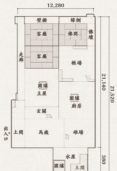
大戶屋 (格局配置圖)
